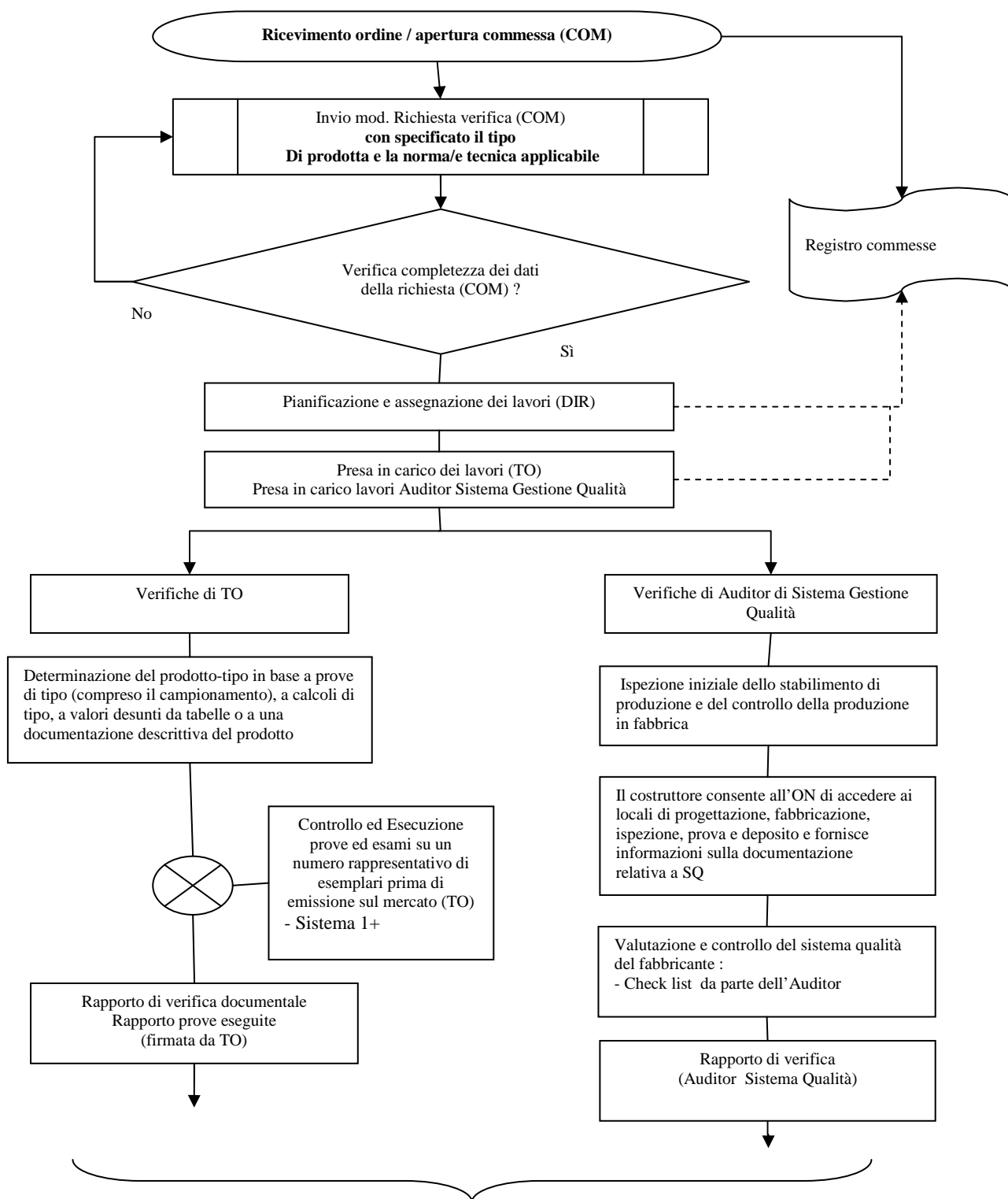
Schema 1-Procedura generale di certificazione della costanza delle prestazioni per i Sistemi 1 e 1+
