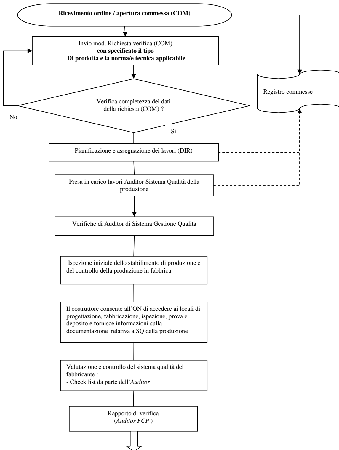
Schema 2 -Procedura generale di certificazione della costanza delle prestazioni per il Sistema 2+
